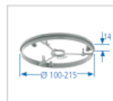
Frontring für das Ortbetonverfahren.
