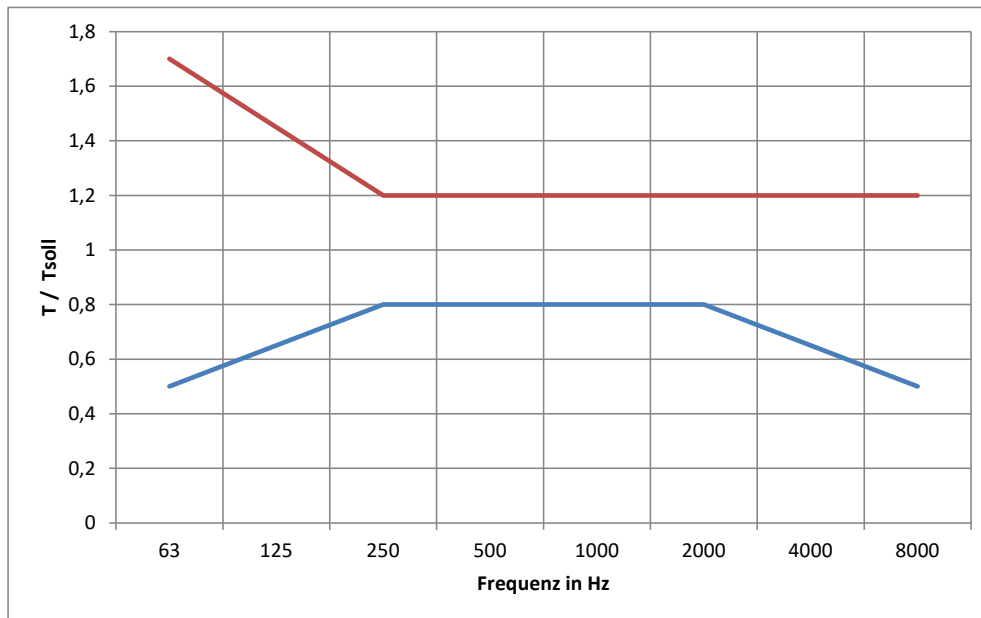
Abbildung 1: frequenzabhängige Nachhallzeit T bezogen auf die Soll-Nachhallzeit
